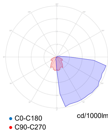
Ljusedistribution: M.I.L Mini
